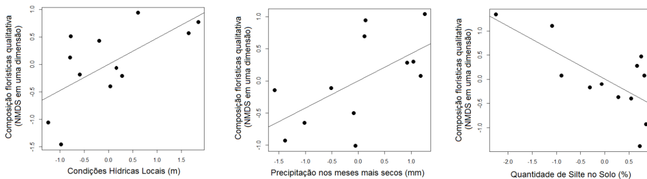
Figura 5. Relações parciais do modelo completo Epa=a+CHL*b1+PMS*b2+SILTE*b3 , onde Epa é o eixo da ordenação com os dados de presença e ausência, CHL são as condições hídricas locais, PMS é a precipitação nos meses secos e SILTE é a porcentagem de silte no solo.
