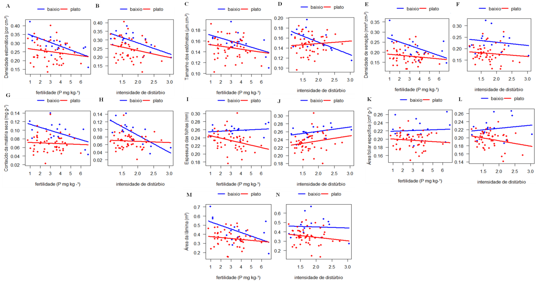
Figura 4: Relação entre a amplitude de variação das características (CV) dentro dos ambientes hidrológicos (baixo e plato) e variáveis ambientais (fertilidade do solo e intensidade de distúrbio). As únicas características que não tem interação com o ambiente são a área foliar específica (K, L) e área da lâmina (M, N) (tabela 5).
