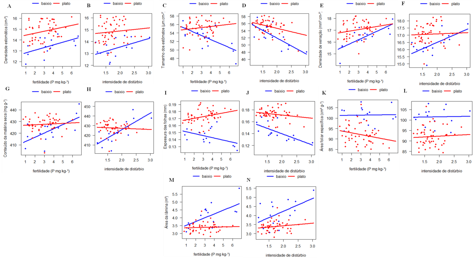
Figura 3: Relação entre valores médios das características funcionais (CWM) e variáveis ambientais (fertilidade do solo e intensidade de distúrbio). A maioria das características teve tendências mais fortes no baixo e a única que não tem interação com o ambiente é a área foliar específica (K, L) (tabela 4).
