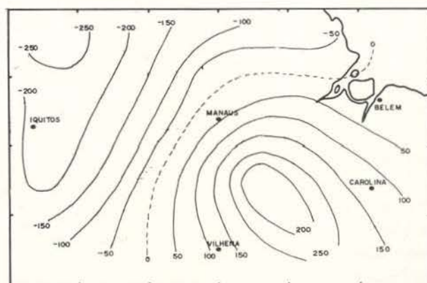
Fig. 7 — Campo da divergência do fluxo de vapor, \nabla \cdot \vec{Q} , para o mês de junho. Média do período 1972/1975. Isolinhhas em mm.
