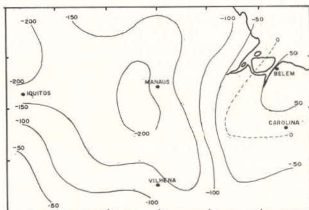
Fig. 6 — Campo da divergência do fluxo de vapor médio, \nabla \cdot \vec{Q} , para março. Média do período 1972/1975. Isolinhhas graduadas em mm.
