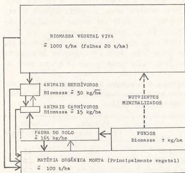
Fig. 2 — Distribuição esquemática da biomassa e fluxo da matéria orgânica no ecossistema de floresta pluvial sobre latossolo amarelo pesado da Amazônia Central (segundo Fittkau & Klinge, 1973).
