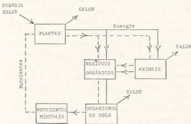
Fig. 1 — Diagrama generalizado de um ecossistema terrestre, mostrando os principais caminhos do fluxo de energia e do ciclo de nutrientes minerais (segundo Richards, 1974).
