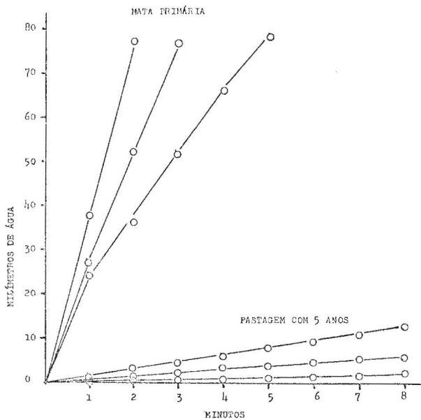
Fig. 3 — Velocidade de infiltração de água no solo nos primeiros minutos de aplicação da água no infiltrômetro, sob mata primária e numa pastagem ao lado, com 5 anos de implantação, latossolo amarelo pesado ao longo da rodovia Manaus-Boa Vista.
